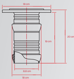
Tubería normal
