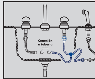
Rociador de Verduras
