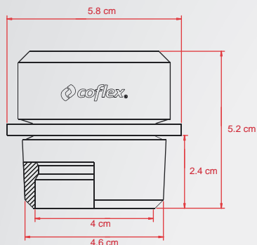
Diseño Industrial MX 43669
